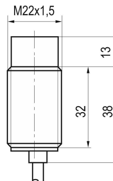
Габаритный чертеж
